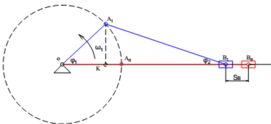
2-rasm. Ichki yonuv dvigatelining krivoship polzun mexanizmi.
